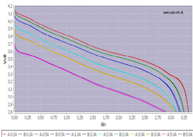
Charakterystyka rozładowania akumulatora XTAR 18650 3500mAh
